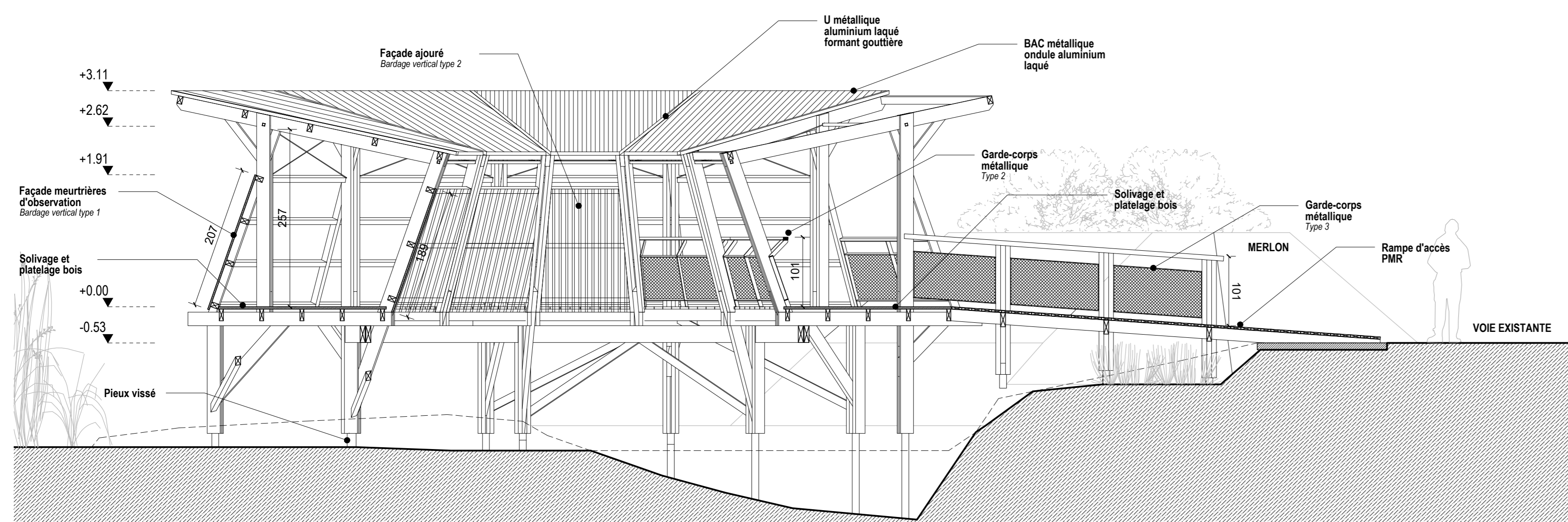
COUPE A-A' ECH 1:50
