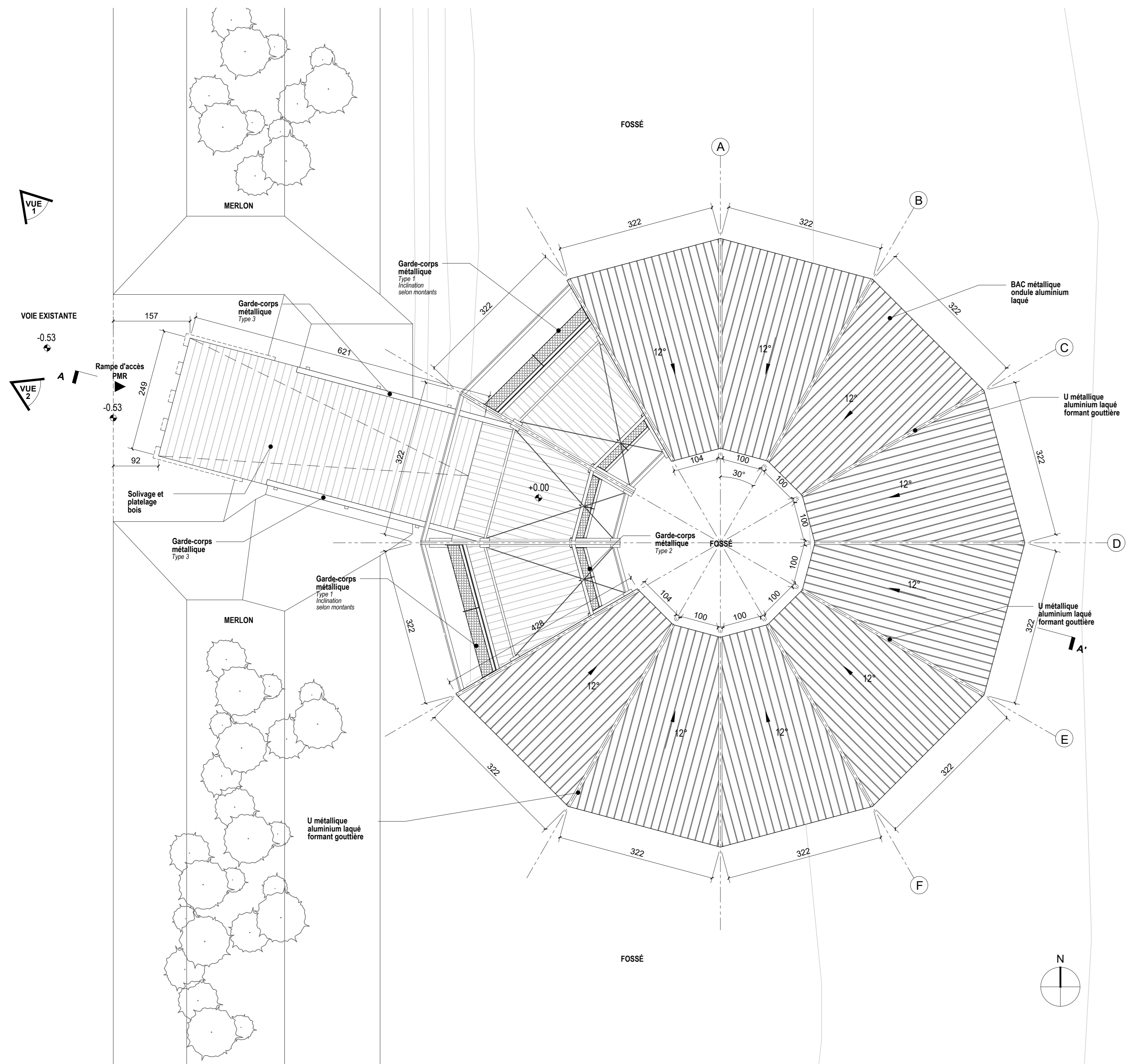
PLAN TOITURE ECH 1:50
