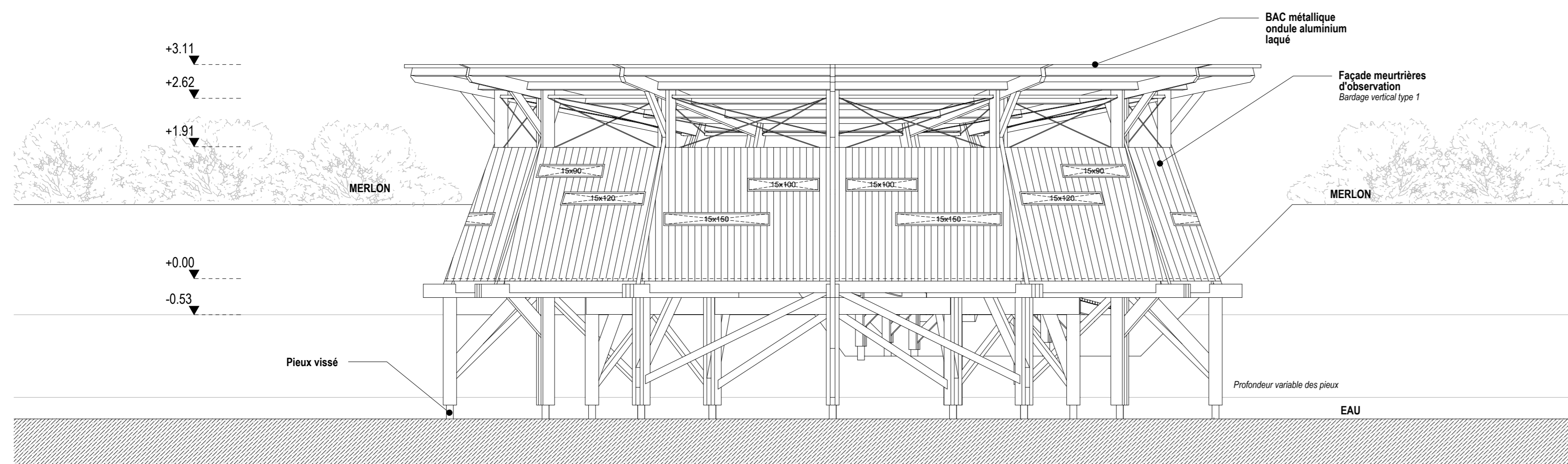
FAÇADE FRONTALE ECH 1:50
